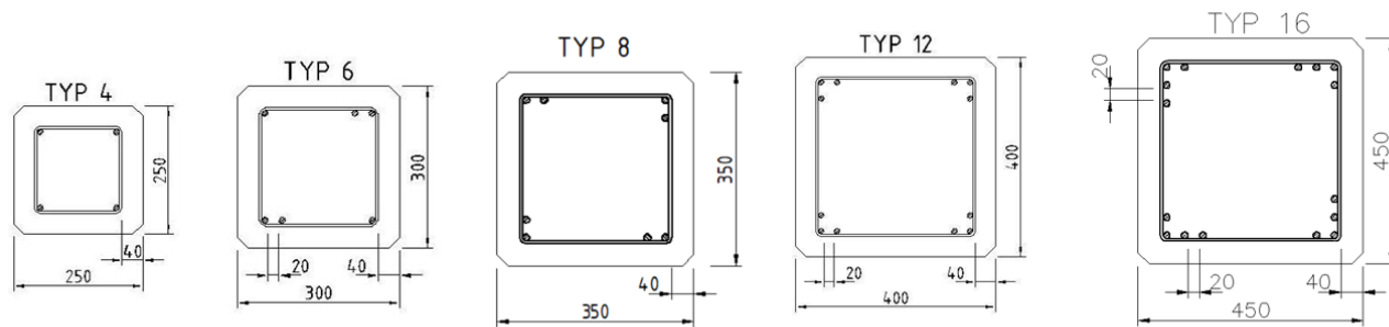
Rysunek 4.2: Typowy układ prętów o średnicy \varnothing 12\text{mm} dla pali 250x250 mm, 300x300 mm, 350x350 mm, 400x400 mm, 450x450 mm
